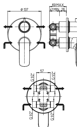
09CR6911 MISCELATORE NOVE DOCCIA INCASSO CON DEVIATORE 2 USCITE KG 1,59 - RB36
