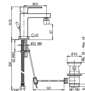
84CR306RS MISCELATORE DAX-R MONOFORO BIDET SCARICO AUTOMATICO 1"1/4 KG 1,53 - RB45
