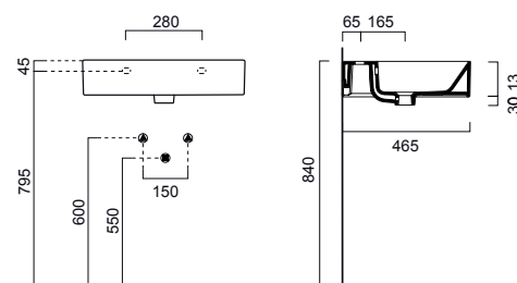
9431111 KUBE BIANCO LUCIDO MONOFORO D'APPOGGIO O A SOSPENSIONE 60X47 - SA279
