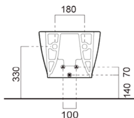
9864111 BIDET MODO SWIRLFLUSH 52X37 SOSPESO - SA271
