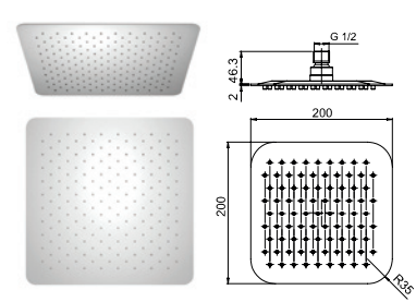
1811054JA00 SOFFIONE CROMO ANTICALCARE IN ACCIAIO INOX 200X200 mm ULTRAPIATTO - RB133
