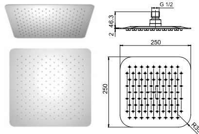
1811055JA00 SOFFIONE CROMO ANTICALCARE IN ACCIAIO INOX 250X250 mm ULTRAPIATTO - RB132
