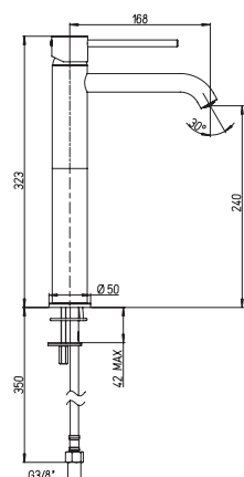
78CR2050LL MISCELATORE COX MONOFORO LAVABO ALTO SENZA SCARICO 1"1/4 KG 2 - RB109
