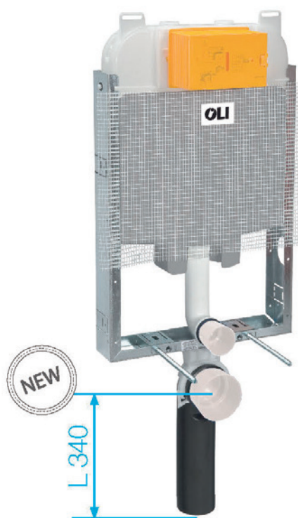
OL0601901 CASSETTA INCASSO OLI 74 PLUS SIMFLEX - SA126
