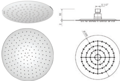
1811053JA00 SOFFIONE CROMO ANTICALCARE IN ACCIAIO INOX DIAM. 300 mm ULTRAPIATTO - RB134
