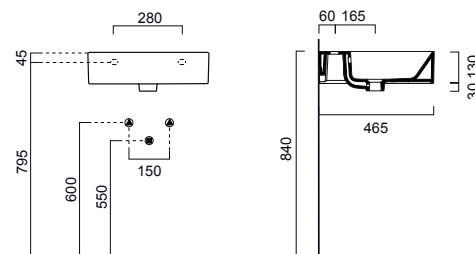
9430111 KUBE BIANCO LUCIDO MONOFORO D'APPOGGIO O A SOSPENSIONE 50X47 - SA278
