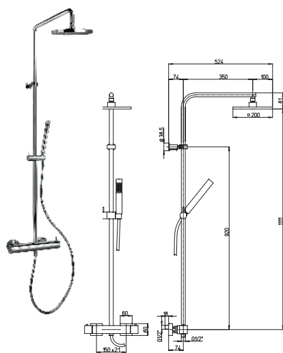
78CR689THAE24P1 COLONNA DOCCIA TONDA TERMOSTATICA con deviatore integrato, maniglie ABS cromate e pulsante di sicurezza 38°, tubi e supporto doccia scorrevole in ottone, soffione ABS Ø 200 mm, doccia anticalcare ABS, KG 5 - RB54
