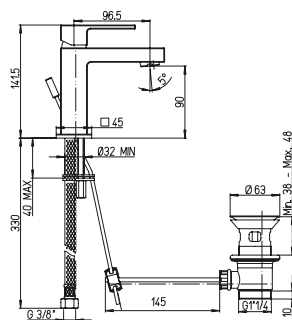
84CR211BLRS MISCELATORE DAX-R MONOFORO LAVABO BOCCA LUNGA SCARICO AUTOMATICO 1"1/4 MEDIO KG 1,8 - RB44
