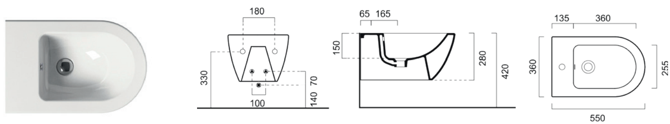
8865111 BIDET SOSPESO PURA BIANCO LUCIDO 55X36 - SA273
