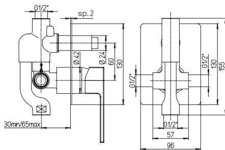
84CR6911R MISCELATORE DAX-R DOCCIA INCASSO CON DEVIATORE ROTATIVO 2 USCITE KG 1,77 - RB47
