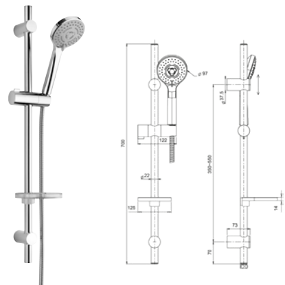
OZU00900JA00 SALISCENDI CROMO ASTA REGOLABILE DIAM. 22 cm 70, DOCCIA 3 GETTI, DIAM. 97 mm, FLESSIBILE cm 150 DOPPIA GRAFFIATURA E PORTASAPONE ISPEZIONABILE - RB150
