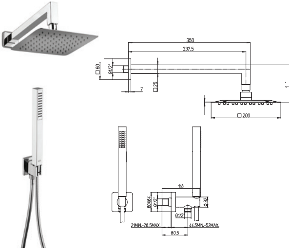
OTW00907JA00 SET QUADRO CROMO COMPOSTO DA SOFFIONE INOX 20X20 cm, BRACCIO, DOCCETTA E SUPPORTO SNODATO CON PRESA D'ACQUA - RB129
