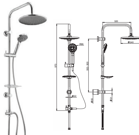
50CR191RSP3 COLONNA DOCCIA TONDA con deviatore e flessibile di collegamento, interasse regolabile, soffione anticalcare ABS 240 mm, doccetta anticalcare ABS 3 getti, tubo acciaio cromato Ø 22 mm, deviatore in ottone, supporto scorrevole ABS, portasapone trasparente, flessibile cromato doppia graffatura cm 150, flessibile di collegamento cm 50 e fissaggi a parete regolabili, KG 2,61 - RB56
