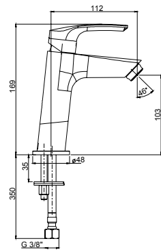
OLU00286JA00 MISCELATORE LUCENTE MONOFORO LAVABO MEDIO SENZA SCARICO - RB124
