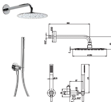
50CR441P4 SET DOCCIA TONDA completo di soffione in Acciaio Inox Ø 250 mm, Braccio da 300 mm con supporto fisso KG 2,5 - RB59
