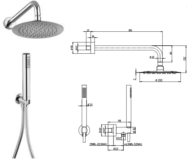
OSU00907JA00 SET TONDO CROMO COMPOSTO DA SOFFIONE INOX DIAM. 20 cm, BRACCIO, DOCCETTA E SUPPORTO SNODATO CON PRESA D'ACQUA - RB130
