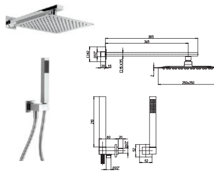
53CR441QQP6 SET DOCCIA QUADRA completo di soffione in Acciaio Inox Ø 250 mm, Braccio da 300 mm con supporto fisso KG 2,9 - RB60
