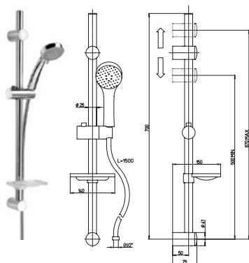
50CR124P1 DOCCIA SALISCENDI P1 con portasapone e doccia anticalcare 3 getti KG 0,99 - RB58
