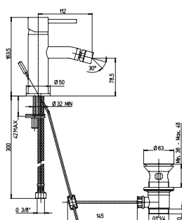
78CR3060 MISCELATORE COX MONOFORO BIDET SCARICO AUTOMATICO 1"1/4 KG 1,64 - RB39
