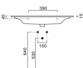
8886111 PURA BIANCO LUCIDO MONOFORO A SOSPENSIONE O SU MOBILI 102X46 - SA277
