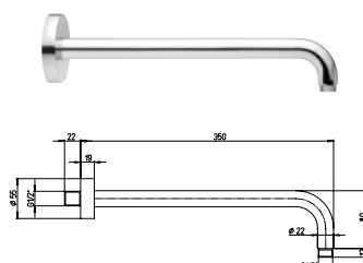
1111073JA00 BRACCIO DOCCIA TONDO CROMO A PARETE DIAM. 22 mm LUNGHEZZA 350mm - RB138
