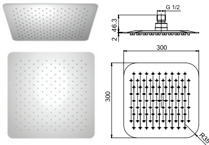
1811056JA00 SOFFIONE CROMO ANTICALCARE IN ACCIAIO INOX 300X300 mm ULTRAPIATTO - RB131
