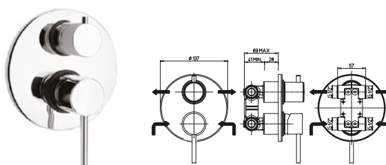
78CR6911 MISCELATORE COX DOCCIA INCASSO CON DEVIATORE ROTATIVO 2 USCITE KG 1,55 - RB41
