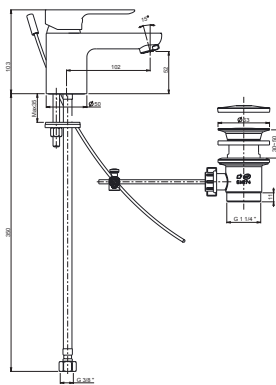
P3CR211 MISCELATORE P3 MONOFORO LAVABO SCARICO AUTOMATICO 1"1/4 KG 1,5 - RB28
