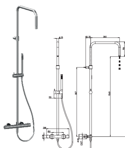
T3CR689TH COLONNA DOCCIA TONDA TERMOSTATICA TRENTA con deviatore integrato, maniglie ABS cromate e pulsante di sicurezza 38°, tubi e supporto doccia scorrevole in ottone, doccia anticalcare ABS, KG 5 - RB144
