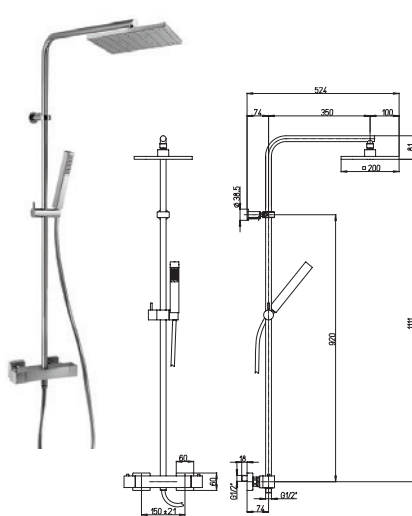
84CR689THE32P1 COLONNA DOCCIA QUADRO ECO TERMOSTATICA con deviatore integrato, tubi e supporto doccia scorrevole in ottone, soffione in ABS quadro 200 mm e doccetta anticalcare in ABS, KG 5,5 - RB55
