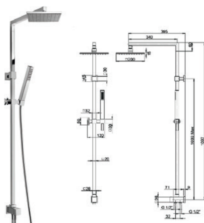
50CR191ARQ4P3 COLONNA DOCCIA QUADRA con deviatore flessibile con col- legamento da 100 cm, interasse regolabile, set di fissaggio in ottone, supporto scorrevole in ottone, flessibile PVC grigio cm 175, deviatore ottone a parete, doccetta anticalcare ABS e soffione in ABS 200 mm, KG 4,5 - RB57
