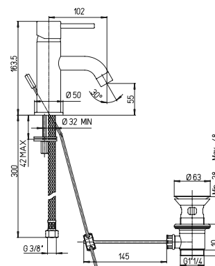
78CR2110 MISCELATORE COX MONOFORO LAVABO SENZA SCARICO 1"1/4 KG 1,7 - RB39
