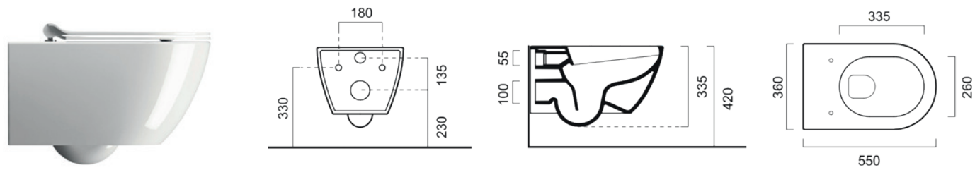
881511 WC PURA SWIRLFLUSH BIANCO LUCIDO 55X36 SOSPESO - SA273
