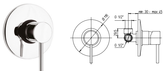
78CR690 MISCELATORE COX DOCCIA INCASSO 1 USCITA KG 0,72 - RB40
