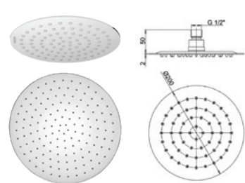
1811051JA00 SOFFIONE CROMO ANTICALCARE IN ACCIAIO INOX DIAM. 200 mm ULTRAPIATTO - RB136
