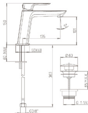
09CR211MESR MISCELATORE NOVE MONOFORO LAVABO BOCCA LUNGA PILETTA CLICK CLACK 1"1/4 KG 2 - RB33
