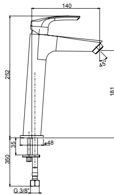
OLU00493JA00 MISCELATORE LUCENTE MONOFORO LAVABO ALTO SENZA SCARICO - RB125
