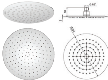
1811052JA00 SOFFIONE CROMO ANTICALCARE IN ACCIAIO INOX DIAM. 250 mm ULTRAPIATTO - RB135
