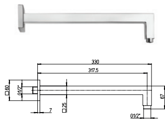
1111008JA00 BRACCIO DOCCIA QUADRO CROMO A PARETE 25X25 mm LUNGHEZZA 330mm - RB137
