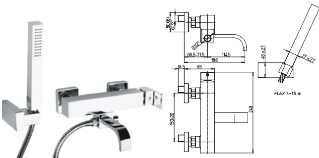
84CR105R MISCELATORE DAX-R VASCA ESTERNO CON DOCCIA DUPLEX KG 3,5 - RB43
