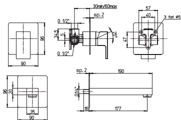
84CR208RQ MISCELATORE DAX-R LAVABO A MURO SENZA PIASTRA KG 1,4 - RB113
