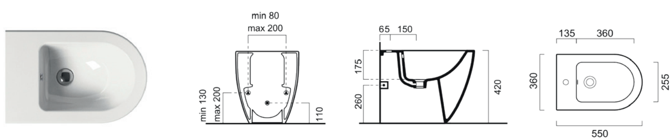
8872111 BIDET MONOFORO PURA BIANCO LUCIDO 55X36 BACK TO WALL - SA273
