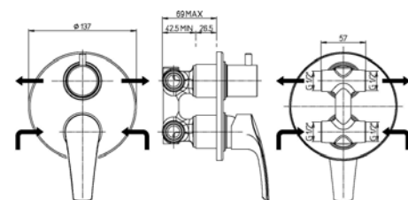
OLU00400JA00 MISCELATORE LUCENTE DOCCIA INCASSO CON DEVIATORE 2 USCITE - RB127
