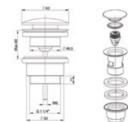
1751051JA01 PILETTA CROMO UNIVERSALE CLICK CLACK TONDA - RB122
